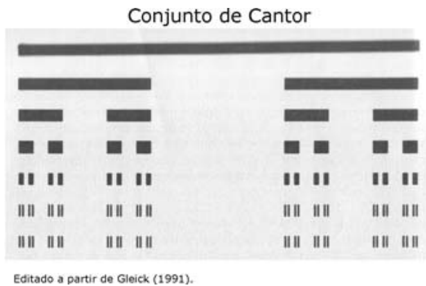
Figura 2.2 - Primeiros sete estágios do processo de construção do Conjunto de Cantor.
