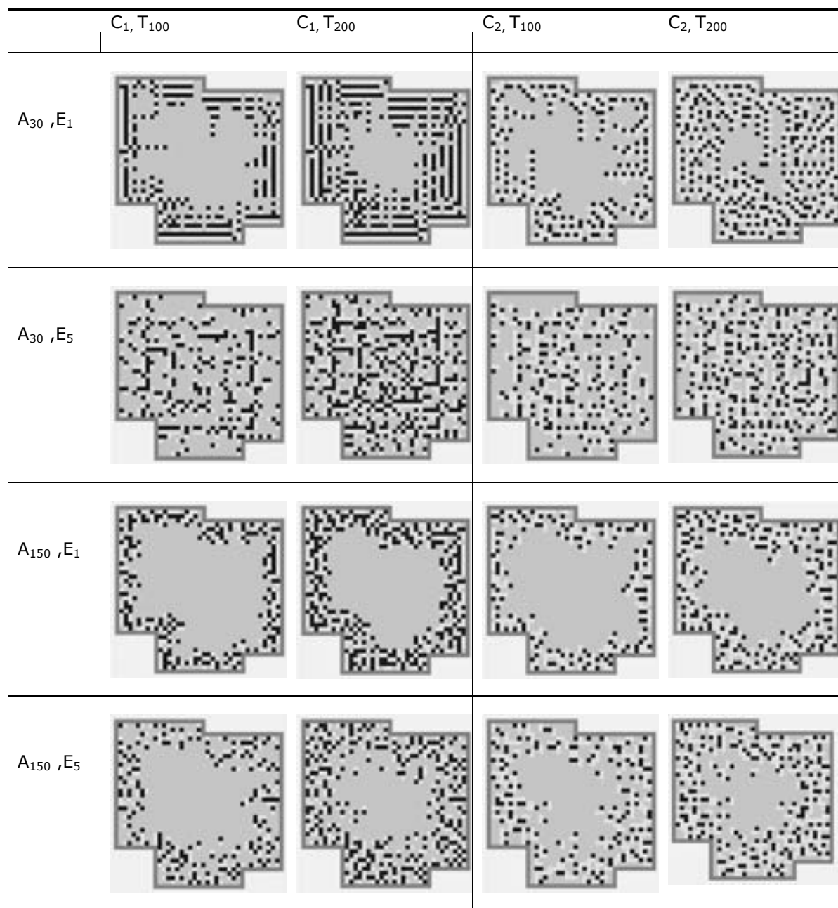
Figura 3.3 - Conjunto de exemplos de padrões morfológicos, gerados a partir de diversas combinações de parâmetros associados aos comportamentos dos agentes no programa FAVELA.
