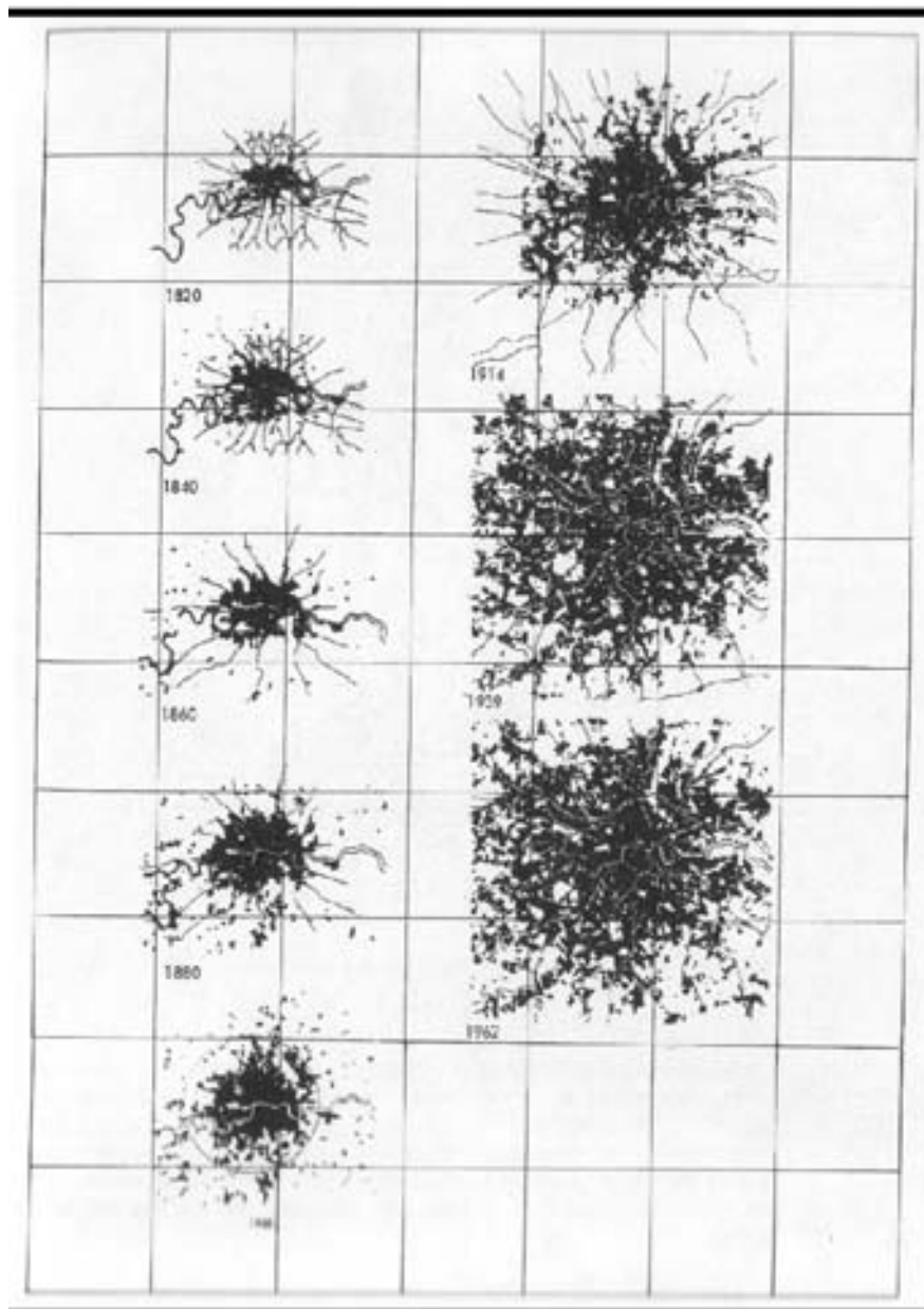
Figura 2.8 - Diversos momentos na evolução da cidade de Londres (Batty e Longley, 1994): 1820, 1840, 1860, 1880, 1900, 1914, 1939 e 1962. Os valores obtidos para a dimensão fractal ( d_m ), neste caso, foram respectivamente: 1.32, 1.58, 1.41, 1.70, 1.73, 1.76, 1.79 e 1.77. Os resultados parecem indicar o mesmo tipo de dinâmica encontrado por Frankhauser para Berlim: a cidade, à medida que cresce, preenche os espaços de forma mais fragmentada e compacta.
